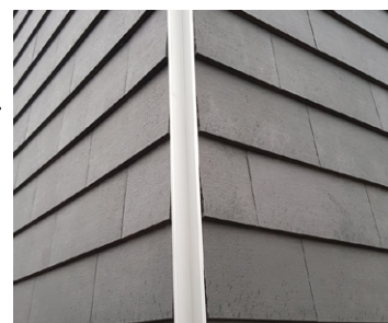
Hjørneløsning med aluminiumsprofil
