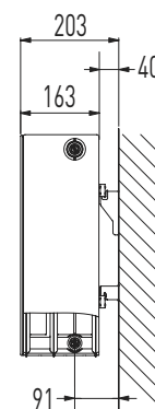
3PK/33, profil
