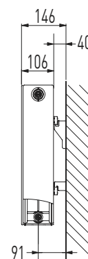
2PK/22, profil
