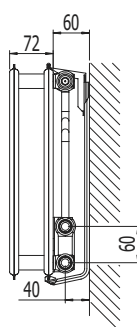
Type 20, profil
