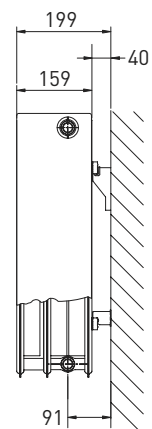
3PK/33-C, profil
