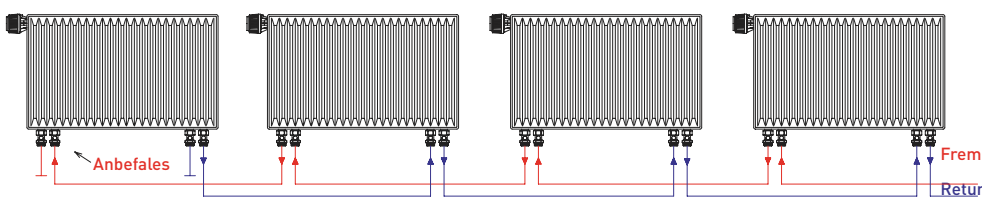
To-strengs ventilsystem
