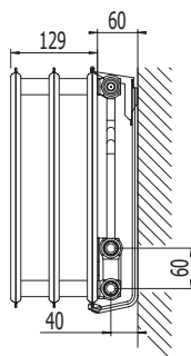
Type 30, profil
