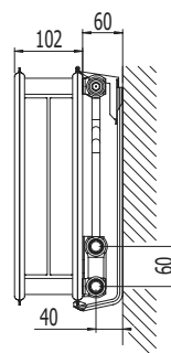
Type 22, profil
