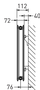
PKP/21, profil
