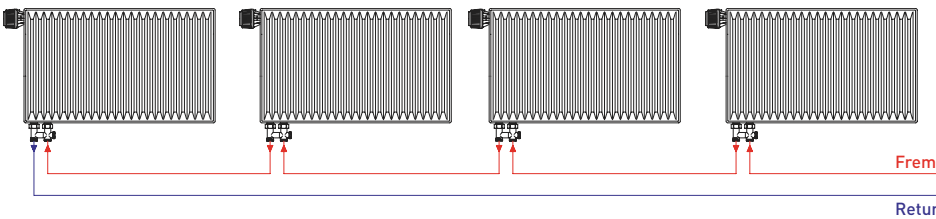
Et-strengs ventilsystem
