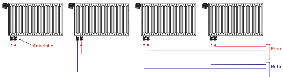
To-strengs ventilsystem
