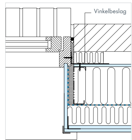
Vinduesmontage i ydervægskonstruktion med skalmur.
