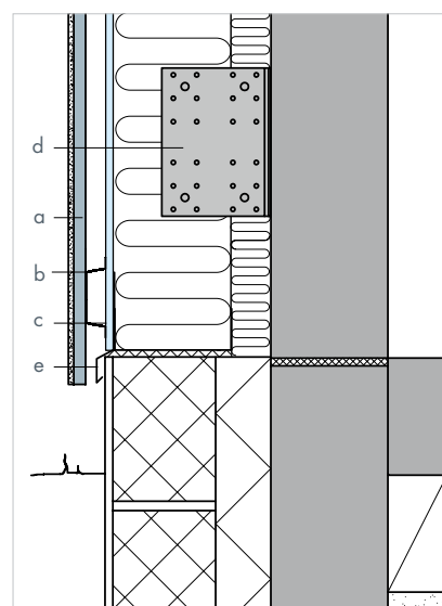
YP12: Fundamenttilslutning
