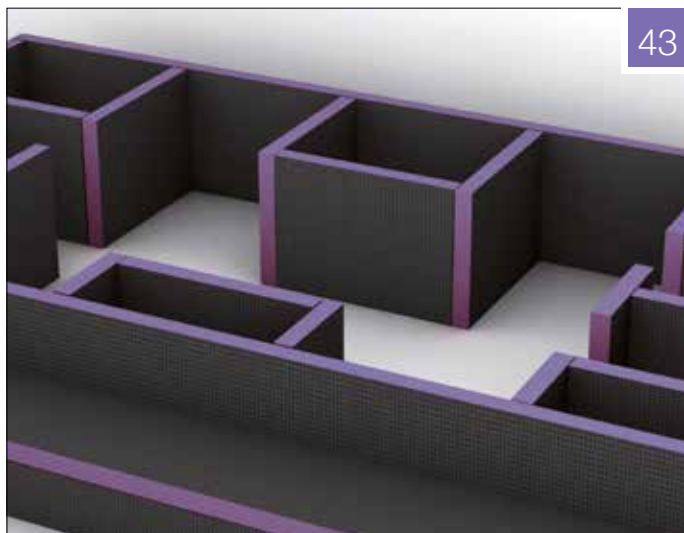
Fig. 43: Mål højden fra gulvet til undersiden af JACKOBOARD® pladen, som skal udgøre toppen af indbygningen.
