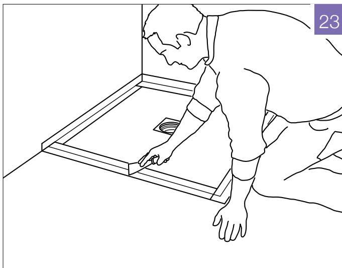
Fig. 23: Forsejl alle samlinger med en godkendt vådrumsmembran.
