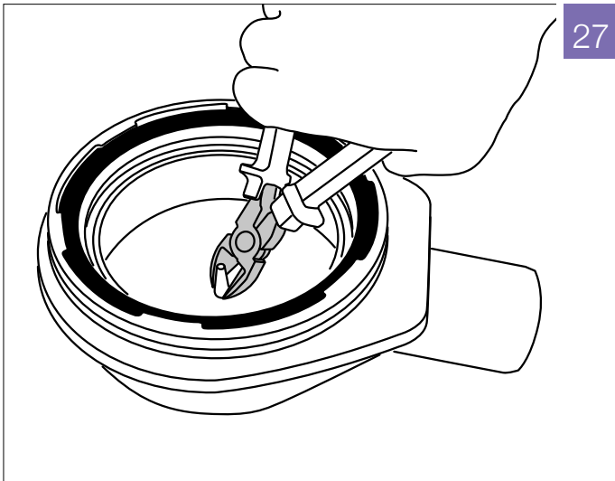
Fig. 27: Plaststiften er ikke nødvendig ved montering af JACKOBOARD® Aqua Line Pro, og skal derfor fjernes.
