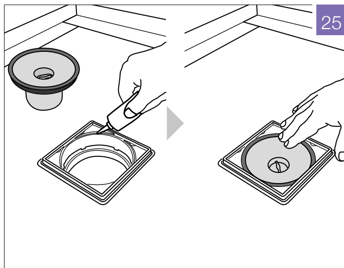
Fig. 25: Smør toppen af rustrammen (8) med armaturfedt. Indsæt derefter vandlåsen (6).
