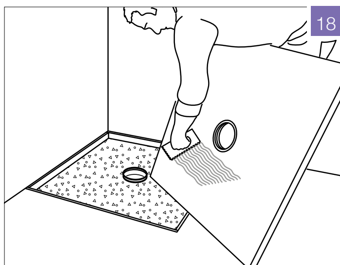
Fig. 18: Når afretningslaget er hærdet, påføres et hurtigtørrende fleksibel cementbaseret fliseklæber på hele undersiden af Aqua elementet (1) med tandspartel.
