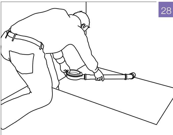
Fig. 28: Tilslut afløbet til det eksisterende DN 50 rør. Placér afløbet nøjagtigt i den rigtige højde. Højdeforskellen mellem den øvre kant af drænrøret og gulvniveauet afhænger af tykkelsen på afløbspladen + 5 mm fliseklæb. (se tegninger side 24).
