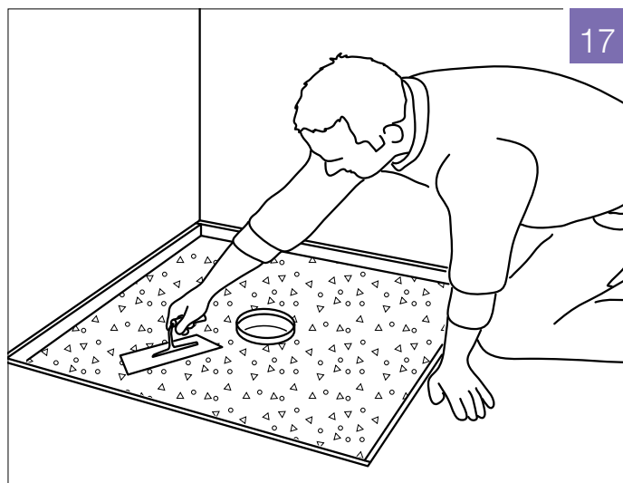
Fig. 17: Udlæg et flydende afretningslag og planér ud til den passende højde. Højdeforskellen til omkringliggende gulvniveau afhænger af Aqua elementets samlede tykkelse inkl. fliseklæber (for yderligere information se side 5).
