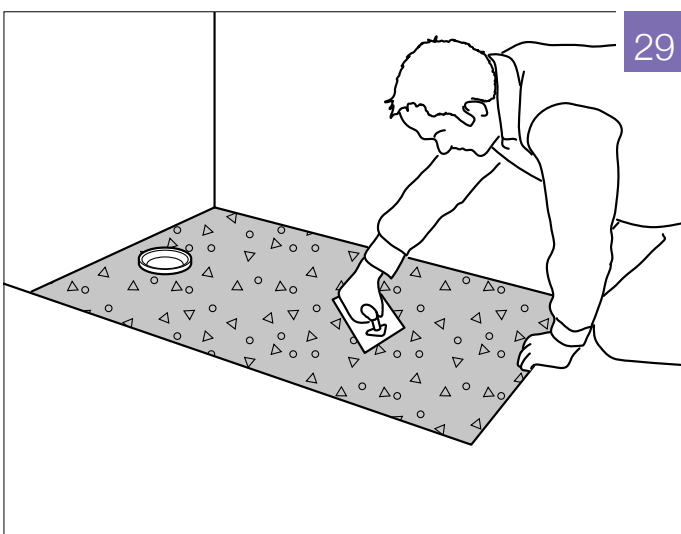
Fig. 29: Udlæg et flydende afretningslag og planér ud til den passende højde. Højdeforskellen til omkringliggende gulvniveau afhænger af afløbspladens samlede tykkelse inkl. fliseklæber (se tegning side 26) Gulvafløbet skal sidde fast i gulvmassen for at kunne absorbere belastning.
