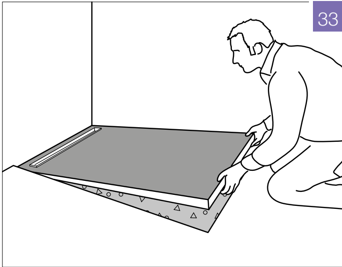
Fig. 33: Anbring forsigtigt JACKOBOARD® Aqua Line Pro i fordybningen, så flangestykket anbringes ned i afløbet.
