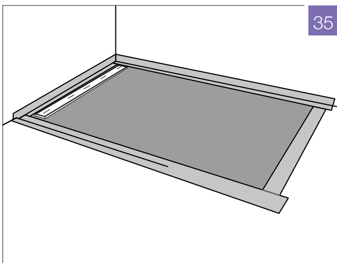
Fig. 35: Installationen af JACKOBOARD® Aqua Line Pro er færdig og elementer er nu klar til påklæbning af fliser.
