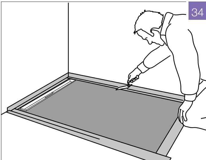
Fig. 34: Forsejl omhyggeligt alle samlinger med en godkendt vådrumsmembran.
