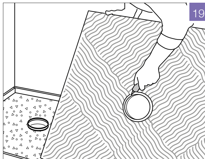
Fig. 19: Smør flangen under Aqua elementet med armaturfedt. Sørg for, at den fabriksmonterede pakningsring er placeret korrekt i afløbet.
