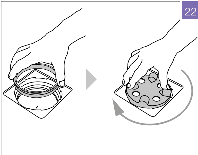
Fig. 22: Indsæt spændekraven (3) - stram det med værktøjet (4).
