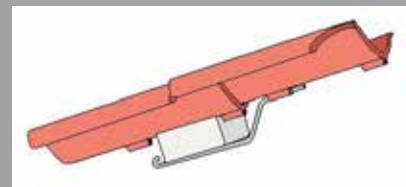
Montering af sidefals binder til HZ 15
