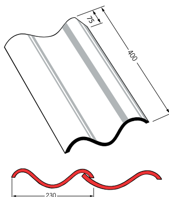
Dobbeltvinge
