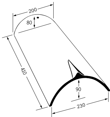
Rygsten 3 stk. pr. lbm.
