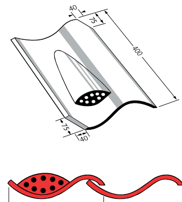
Ventilationssten
