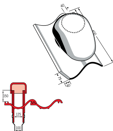
Lodret tudsten Ø 100 til 125 mm
