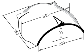
Start rygsten til valm
