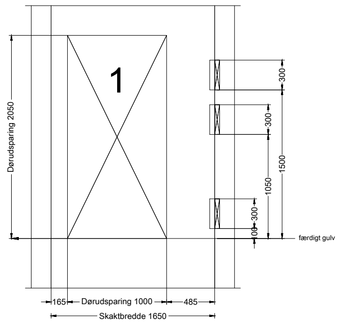
Betonlysning Etage (1)
