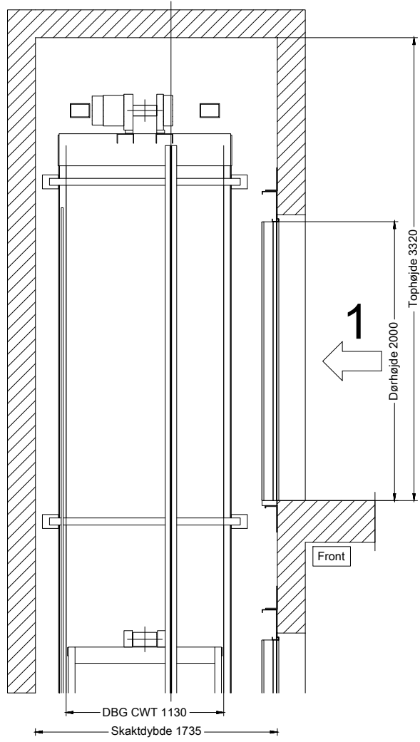
Tværsnit
