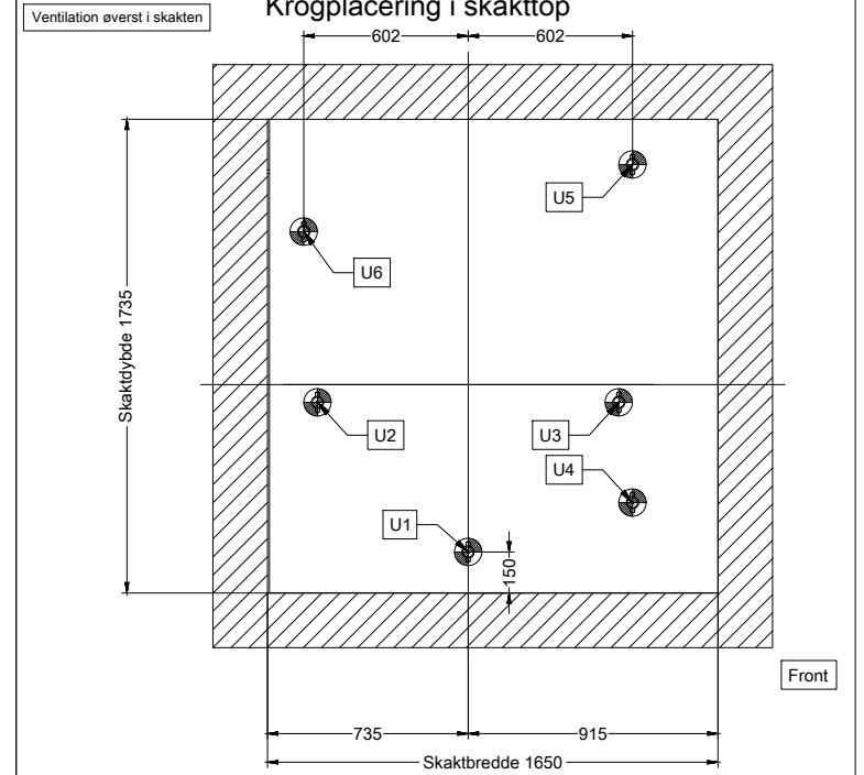
Plansnit Krogplacering i skakttop
