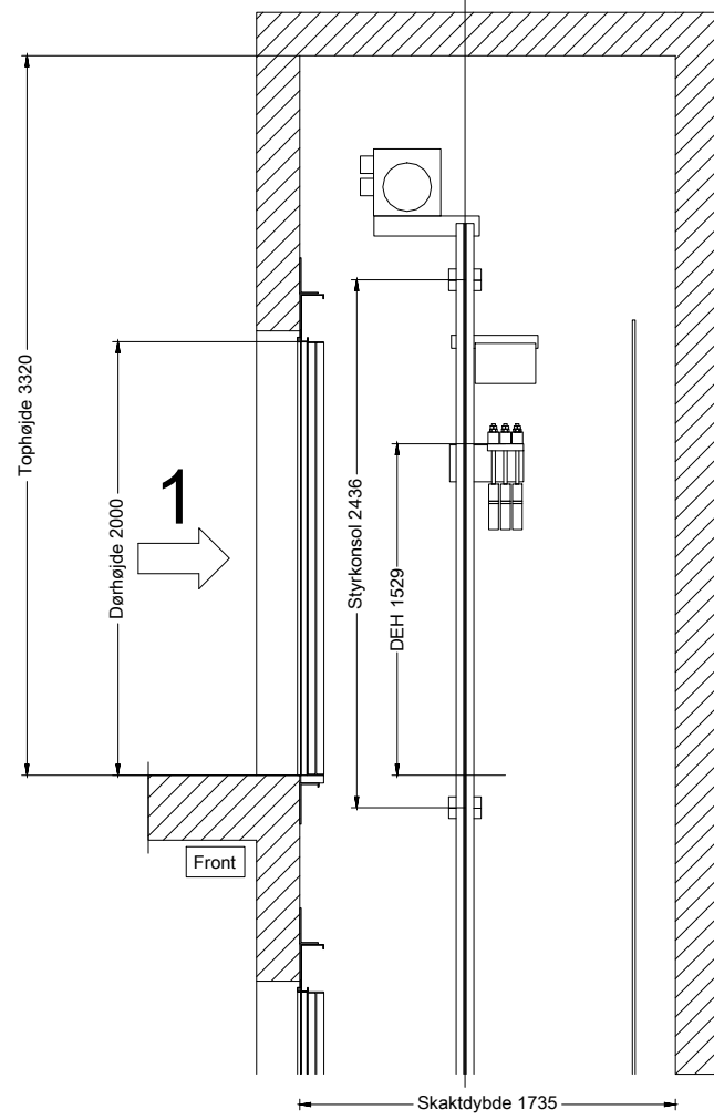
Tværsnit
