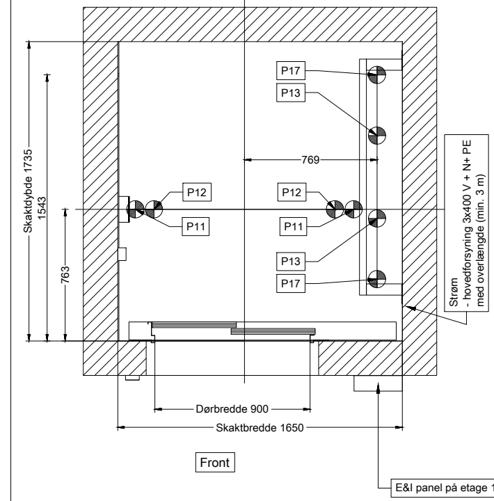
Plansnit Etage 1 Reaktioner i grubebund
