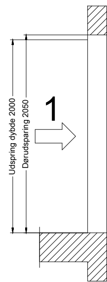
Betonlysning (1)
