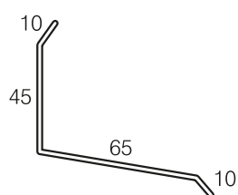
Murinddækning til Fastlock
