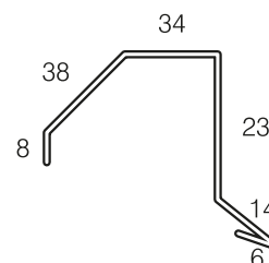
Sterninddækningsprofil til Fastlock
