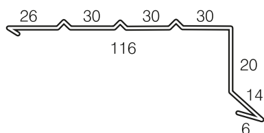
Universalkapsel til Fastlock
