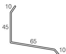
Facadeinddækningsprofil til Fastlock
