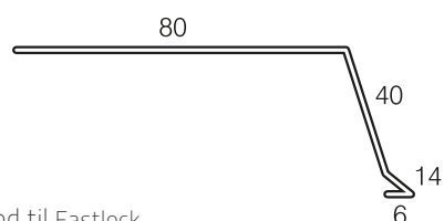
Tagfod til Fastlock
