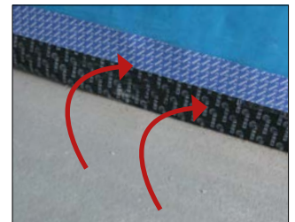
Det er vigtigt, at sokkel- og remfolien altid klæbes opad fast underlaget
