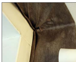
Ved betonvægge fastgøres lysningsfoliens butylklæber til betonfalsen. Samlingen trykkes med en trykrulle. Det skal sikres, at butylen klæber til underlaget.
