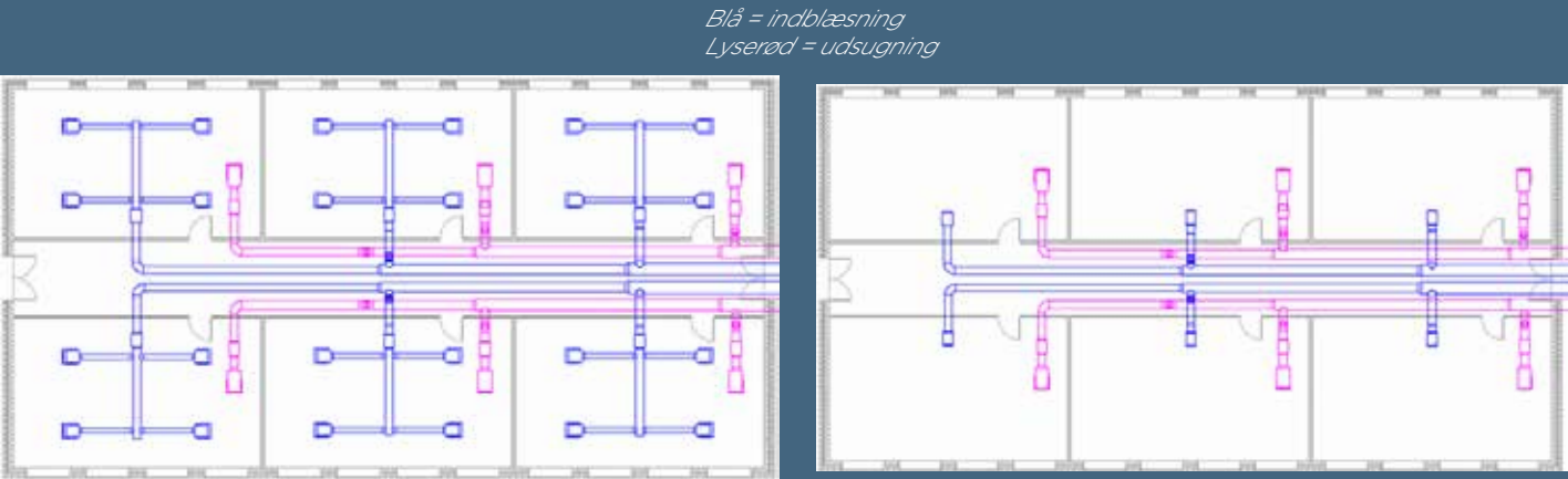
Plantegning af ventilationskanaler til 6 klasselokaler med traditionel ventilation
