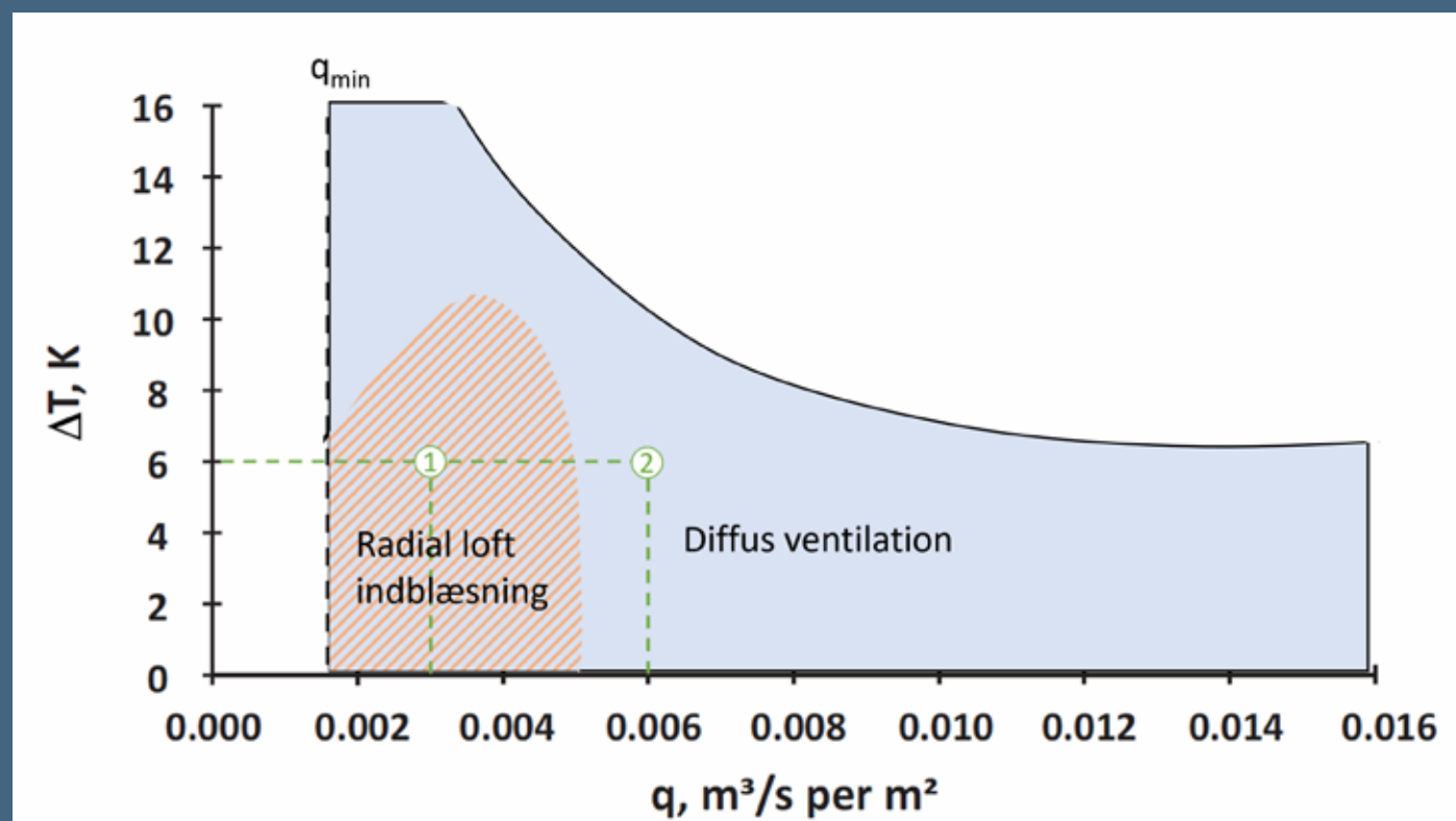
FIGUR 2: Q-T DESIGNCHART FOR KOMFORT VED VENTILATION
